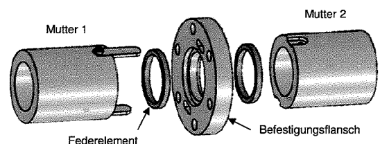
Abbildung 1: Schematische Darstellung der Doppelmutter
