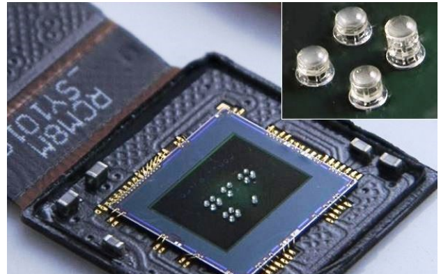
Abbildung: CMOS-Sensor mit mehreren direkt aufgedruckten Arrays von je vier Linsen-Systemen unterschiedlicher Brennweite [Bild: Universität Stuttgart].
