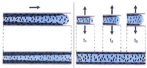
Abbildung: Vergleich der resultierenden Füllstofforientierung zwischen herkömmlichem Spritzgießverfahren (li.) und erfindungsgemäsem Zusatzhub (re.). Das Verhältnis von Kernschicht (blau) zu Randschicht (grau) wird deutlich erhöht und eine zuvor nur selten auftretende senkrechte Orientierung einzelner Partikel (li.) wird durch die Hubbewegung des Werkzeugs (re.) deutlich verstärkt [Bild v.n. Uni Stuttgart].
