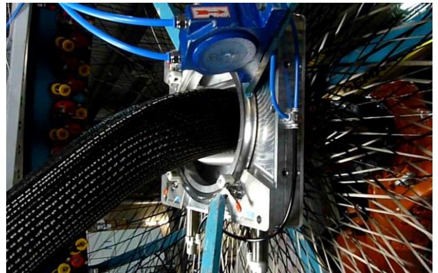
Abbildung: Anpresswalzenmechanismus integriert in eine Radialflechtmaschine.
