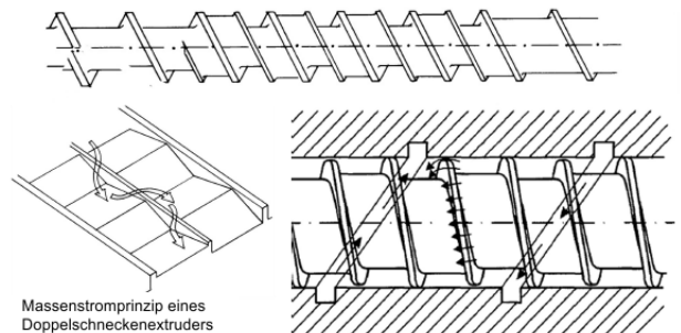
Abbildung: Massendurchsatz durch den genuteten Zylinder in Kombination mit einer Wellenschnecke.
