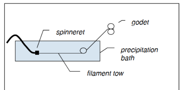
Abbildung 2: Schema des Direktspinnverfahrens: Die in einer ionischen Spinnlösung aufgelöste Cellulose wird durch die Mikrolöcher einer speziellen Spinnöse gepresst und im Fällbad zur Faser koaguliert und gezogen. Die Fasern können als Stapelfasern oder aufgewickelt als Endlosgarn gelagert und verarbeitet werden.
