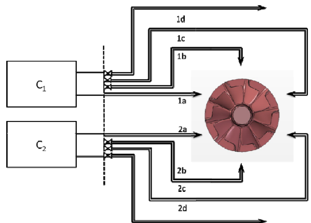
Abbildung 1: Prinzip der Erfindung am Beispiel eines Zweizylindermotors
